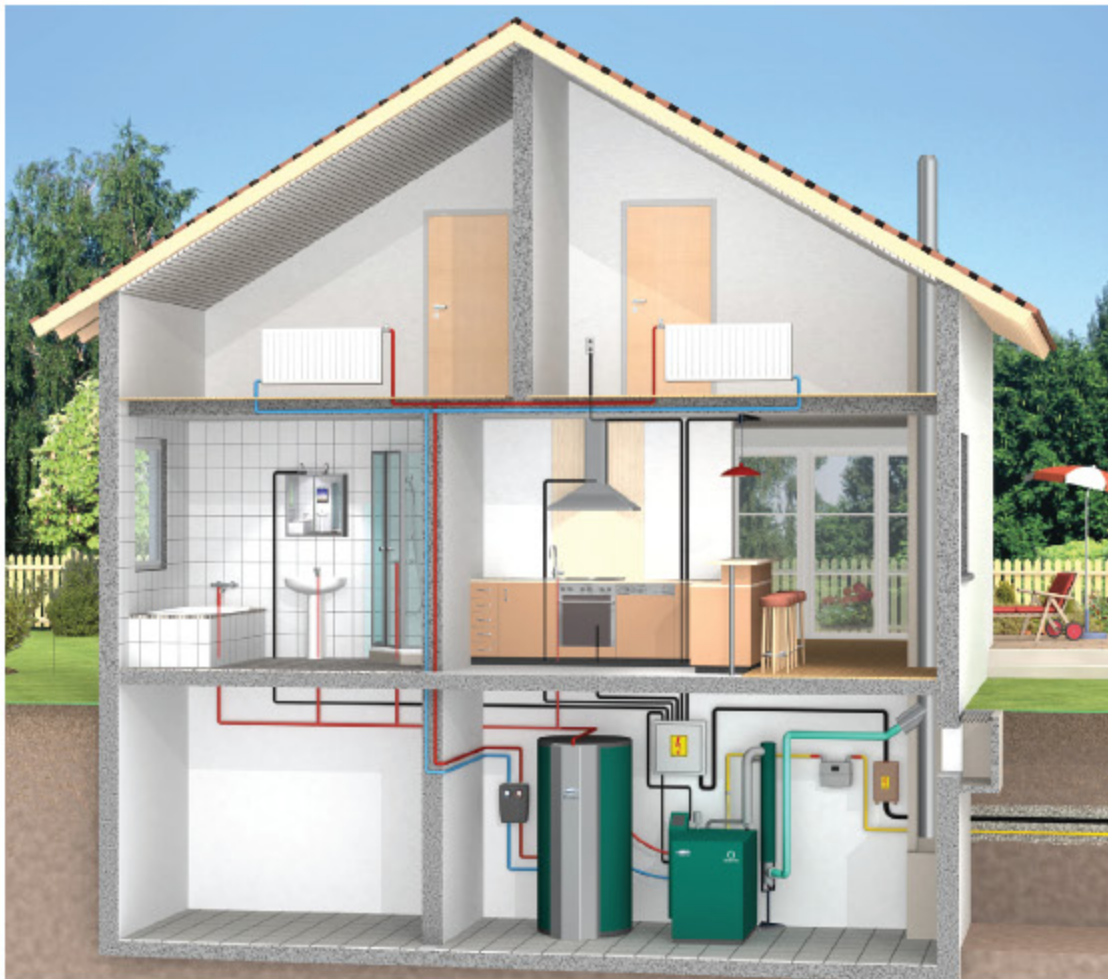
Elektrische und heizungstechnische Einbindung im Ein- und Mehrfamilienhaus mit dem Dachs SE
